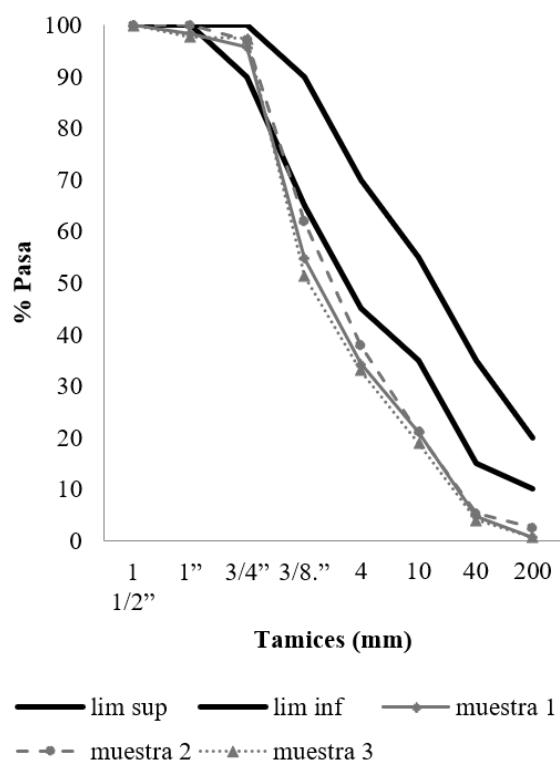
Figura 3. Curva granulométrica.
